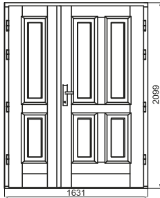
DOUBLE DOOR asymmetrical Lhotse
